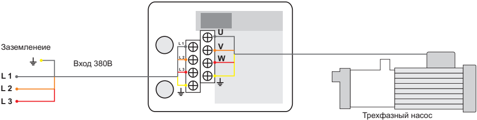
Схема подключения
